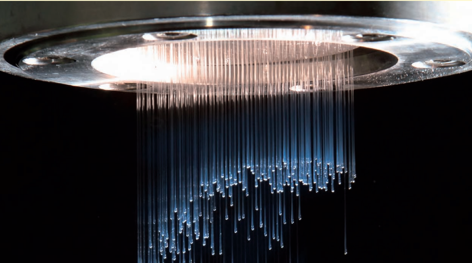
Trockenspinnverfahren mit Keramikfasern.
