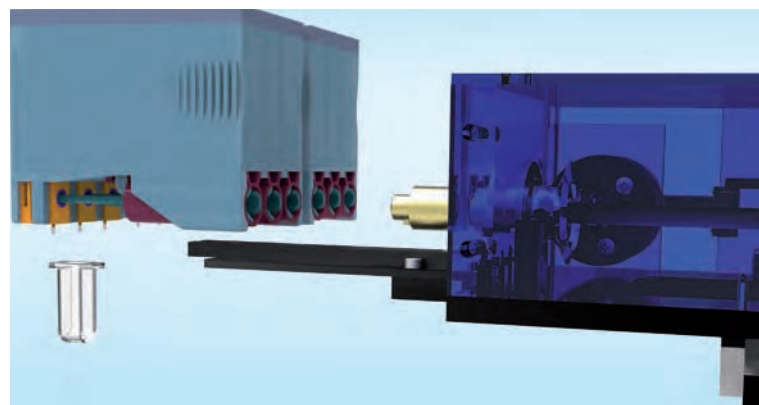
Illustration einer Reagenzkartusche mit integriertem Dispenser und externem Aktuator.
