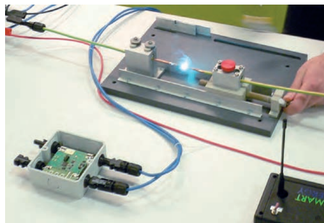
Die Funksensorik erkennt Lichtbögen.
