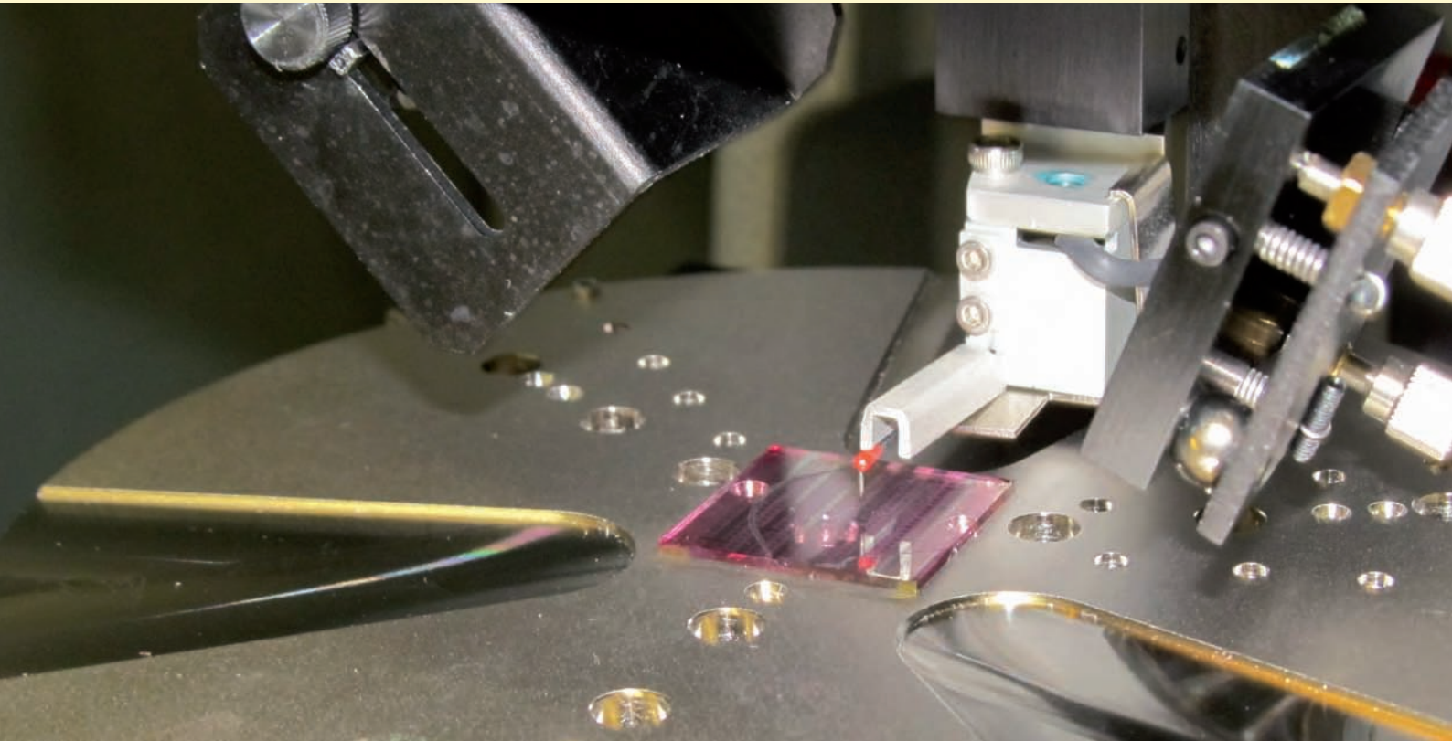
Schichtcharakterisierung an gedruckten, organischen Feldeffekttransistoren (OFET) mittels eines (Dektak-)Profilometers.
