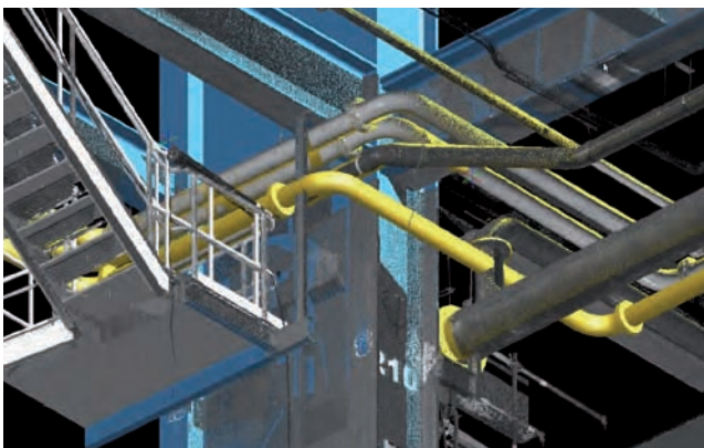
Kombinierte Darstellung von Bestand (Laserscan-Punktwolke) und Neuplanung.
