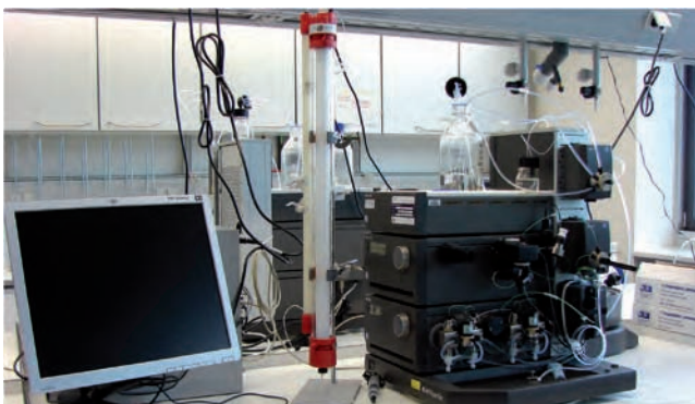
Chromatographieranlage zur „klassischen“ Aufreinigung von Proteinen. Neben dem Pumpensystem (rechts) und der Computersteuerung sind zwei Trennsäulen zu sehen.
